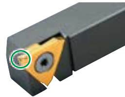
Groove width 1.0mm
